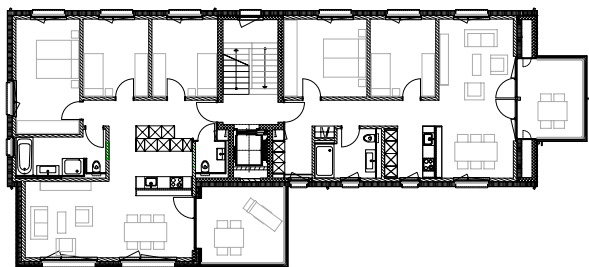
2. Obergeschoss
